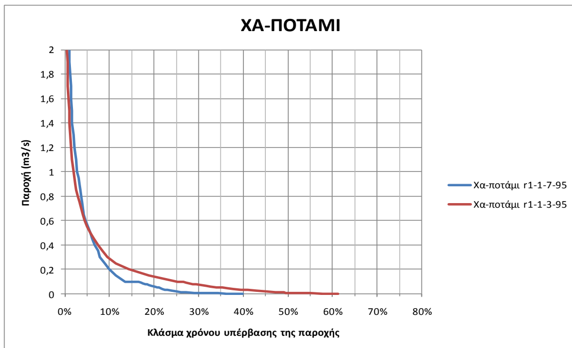
Σχήμα 8-12: Σχέση παροχής-διάρκειας
