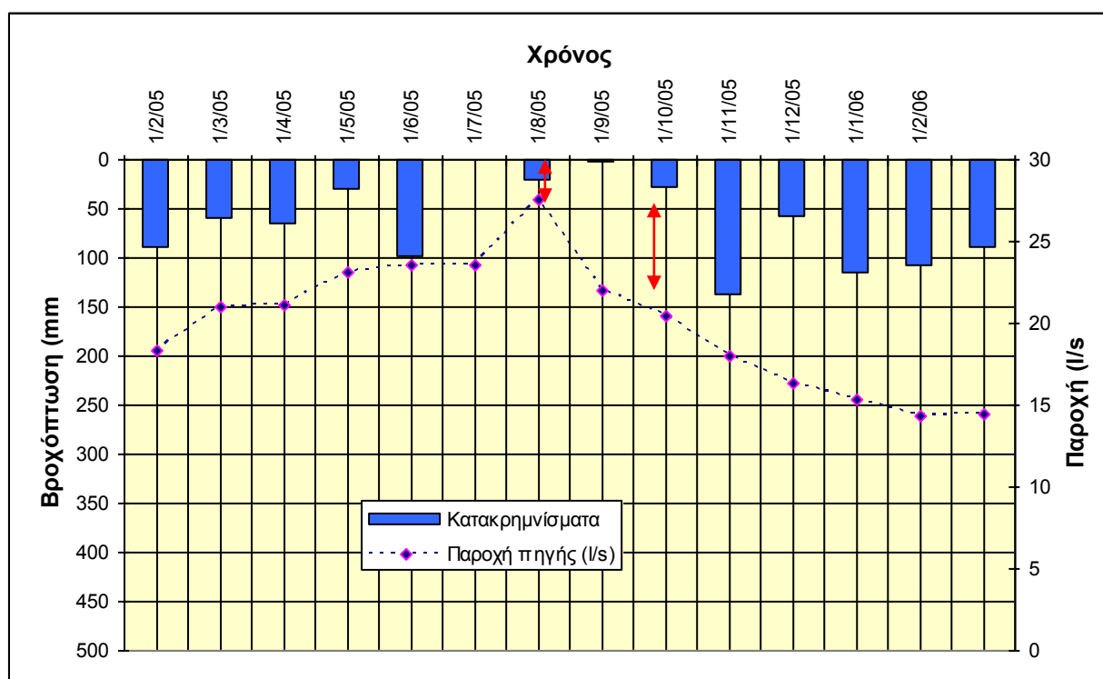
Σχήμα 8-6: Επίδραση μεμονωμένων επεισοδίων υετού στην μορφή του υδρογραφήματος (πιθανόν λόγω μεθοδολογίας μετρήσεων) στην πηγή Αρκολαχανιά
