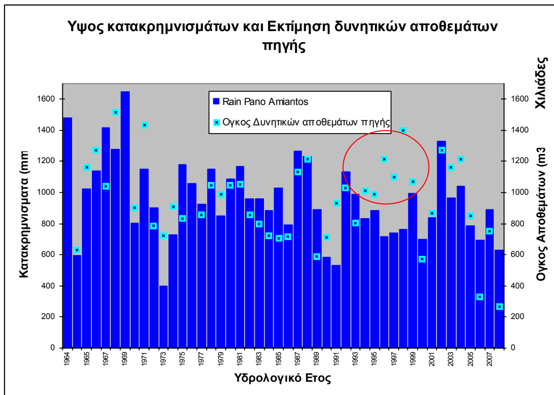
Σχήμα 8-7: Εκτίμηση δυνητικών αποθεμάτων πηγής s9-6-3-50 (ARKOLAKHANIA) και ετήσιο ύψος κατακρημνισμάτων ανάντη της πηγής σταθμού (Πάνω Αμιάντος). Υπογραμμίζεται χρονική περιοχή με αμφίβολα αποτελέσματα
