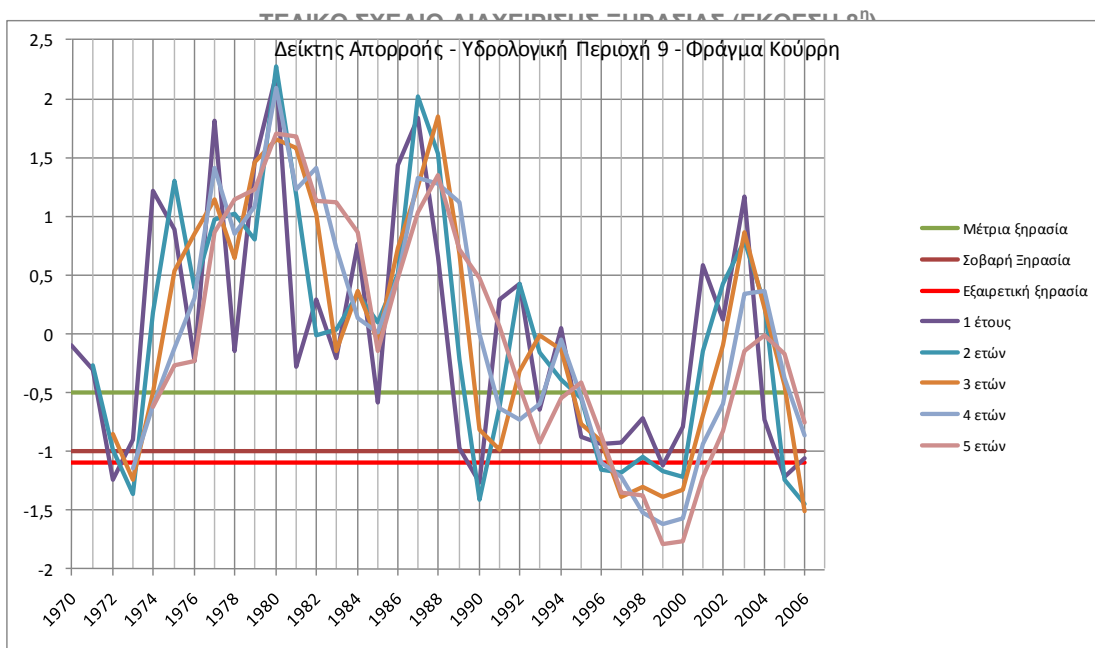
Σχήμα 2-14: Σύγκριση Δεικτών Απορροής Υδρολογικής Περιοχής 9
