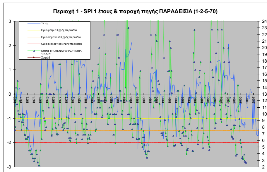
Σχήμα 2-23: Παροχή Πηγής και Δείκτης Ξηρασίας (SPI) – Υδρολογική Περιοχή 1
