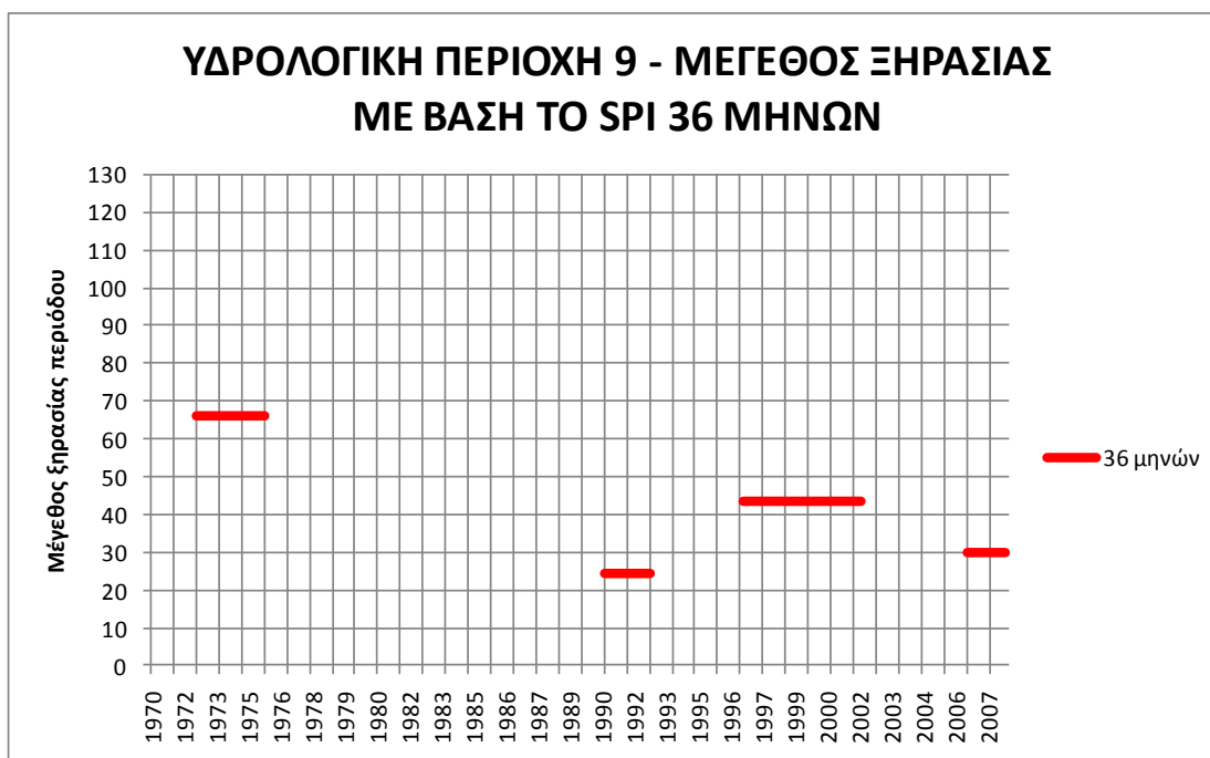
Σχήμα 2-4: Μεγέθη Ξηρασίας της Υδρολογικής Περιοχής 9 για SPI 36 μηνών
