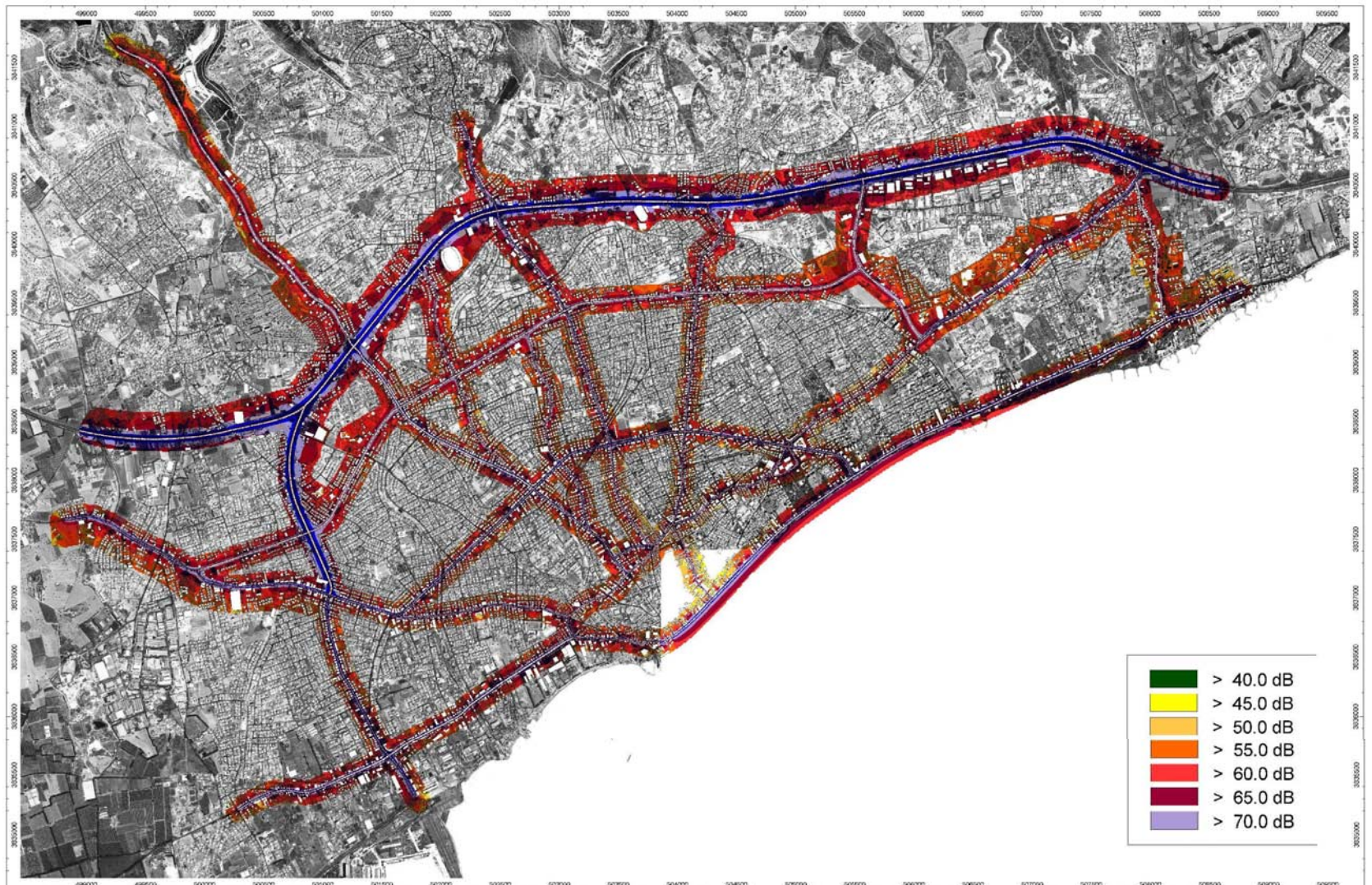
ΣΧΘ Λεμεσού - Δείκτης Lden 2007
